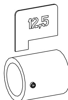
G Bague de réglage et entretoise 12,5 Brûleur vertical - Droit
